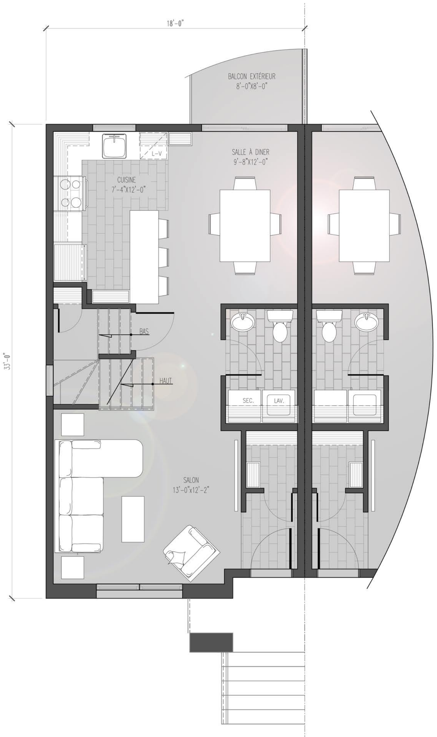
REZ-DE-CHAUSSÉE (580 pi2)
